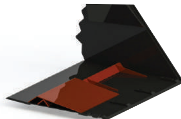
Двойное основание «челюсти», продольное и поперечное усиление
