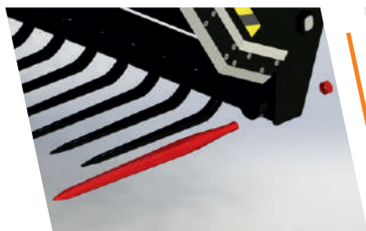
Усиленные боковые пики
